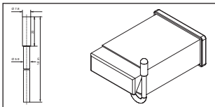
Abb. 2: Montage mit gekürztem Fühler Fig. 2: Assembly with shortened sensor Fig. 2: Montage avec sonde raccourcie Afb. 2: Montage med ingekortet sensor Bild 2: Montaggio con sonda a misura Imagen 2: Montaje con sensor recortado 図 2: 短くしたプローブの取付け
