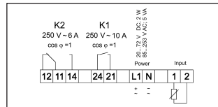
Abb. 3: Anschlusssschema Fig. 3: Connection diagram Fig. 3: Schema de connexion Afb. 3: Aansluitschema Bild 3: Anslutningsschema Fig. 3: Schema d'alimentazione Imagen 3: Esquema de conexión 図 3: 結線図
