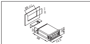
Abb. 1: Gerätermontage Fig. 1: Assembly Fig. 1: Montage de l'appareil Afb. 1: Apparatmontage Bild 1: Aggregatmontage Fig. 1: Montaggio dell'apparecchio Imagen 1: Montaje del aparato 図 1: 組立
