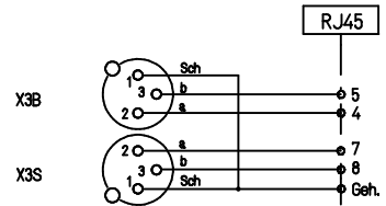
Riedel Belegung Modul XLR Buchse/Stecker > RJ45
