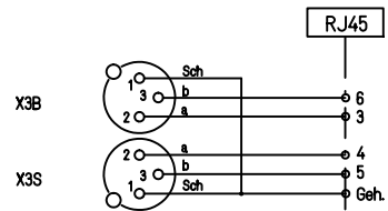
Clearcom Belegung Modul XLR Buchse/Stecker > RJ45
